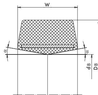
km = konischer Reifenfuß/ conical base tyre/ bandage à base conique mittengeteilt (symmetrisch)/ centre split (symmetrical)/ partagé centralement (symétrique) km 15 = \alpha 15° km 8 = \alpha 8°
