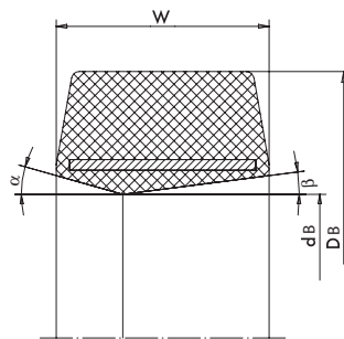
ks = konischer Reifenfuß/ conical base tyre/ bandage à base conique seitengeteilt (asymmetrisch)/ laterally split (asymmetrical)/ partagé latéralement (asymétrique) ks 15/6 = \alpha 15°, \beta 6° ks 23/9 = \alpha 23°, \beta 9°
